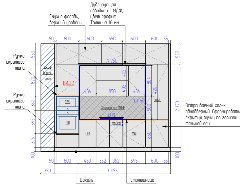
Схема 1. Кухонный гарнитур
