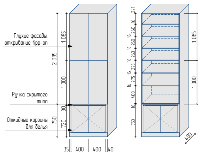
СХЕМА 1. Основные размеры шкафа
