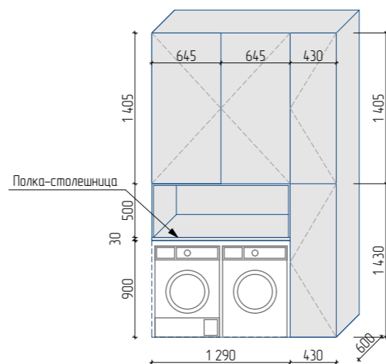
СХЕМА 2. Основные размеры хоз. шкафа
