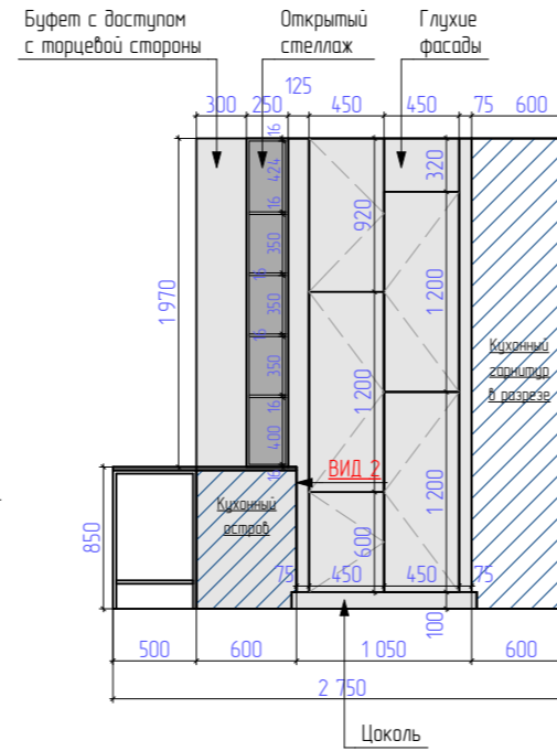
Вид 1. Кухонный шкаф
