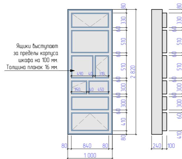
Схема 4. Стеллаж
