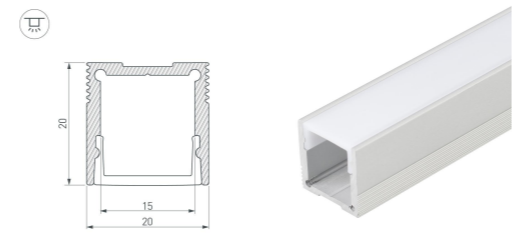
Схема 2. Профиль SL-SLIM20-H20-2000 ANOD, Артикул 023722. Крепление произвести вровень с рейками 20x20
