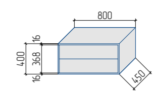
СХЕМА 2. Основные размеры прикроватной тумбы
