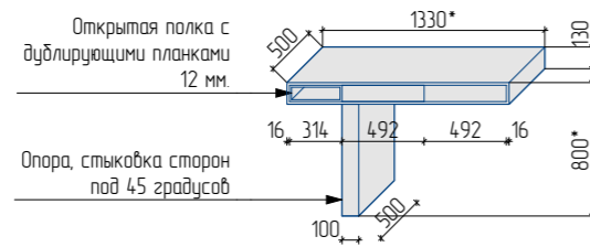
СХЕМА 1. Основные размеры стола
