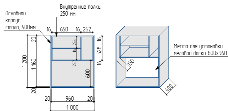
Основные размеры стола
