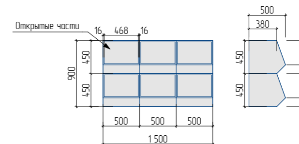
Основные размеры системы хранения для игрушек
