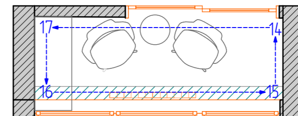
ПЛАН РАЗВЕРТОК
