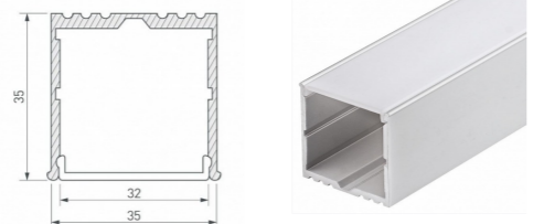
Схема 1. Профиль ARH-POWER-W35-2000 ANOD, Артикул 016138. Крепление произвести вровень с МДФ панелями и зеркалом
